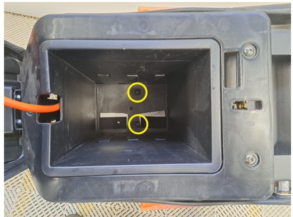
Irrota akkulaatikon kaksi kiinnityspulttia. (kuusiokoloavain 5 mm).
