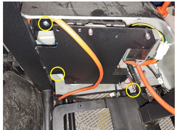
Irrota vasemmanpuolen kylkipaneelin kolme kiinnitysruuvia. (ristipäämeisseli ph2).
